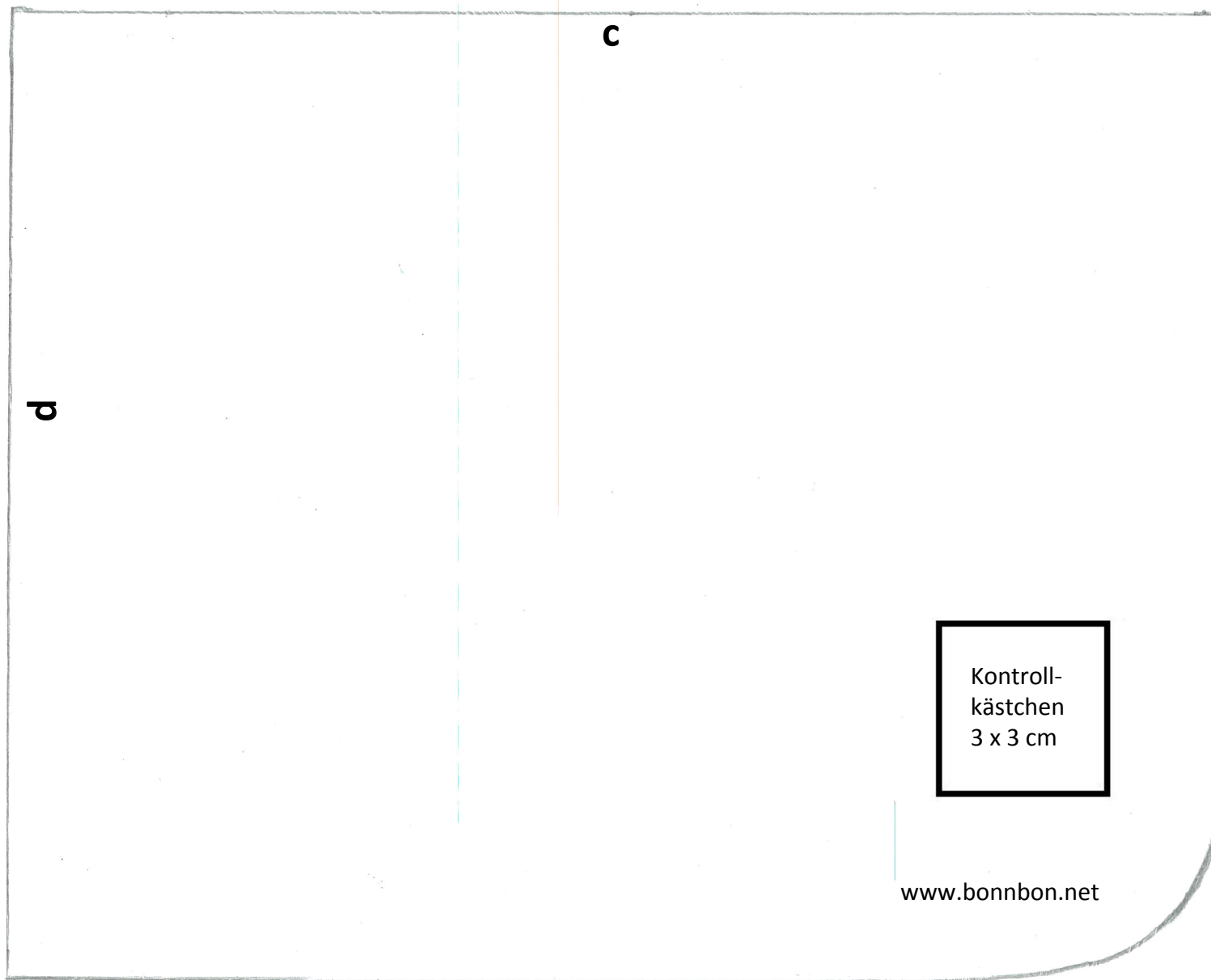
Schnitt: Seitenteil Picknicktasche
