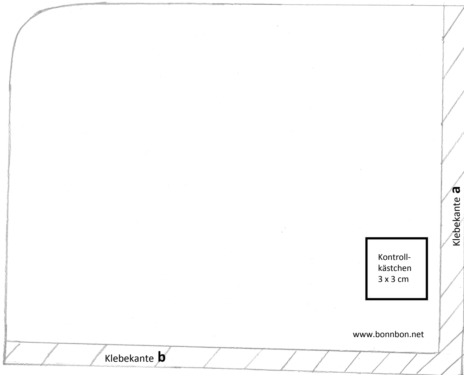
Schnitt: Seitenteil Picknicktasche
